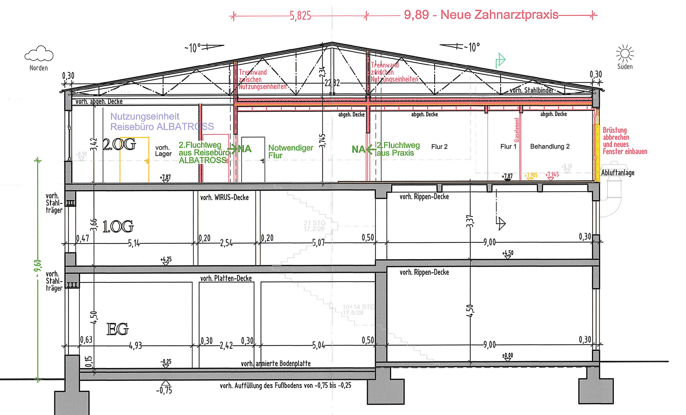
Querschnitt M 1:100
