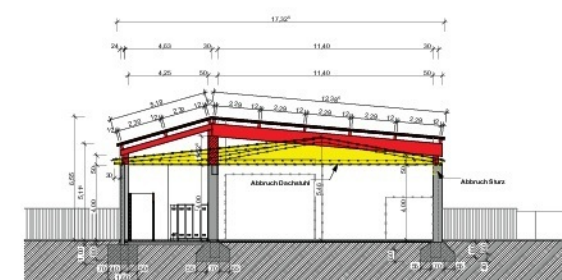
ABBRUCH/NEUBAU SCHNITT S-01
