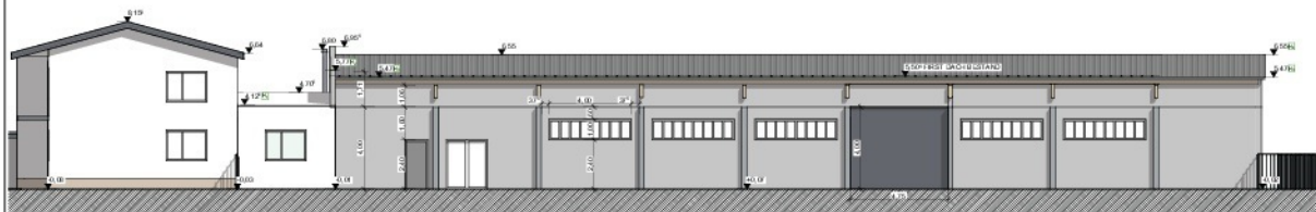
ENDZUSTAND ANSICHT A-02 NORD-OST
