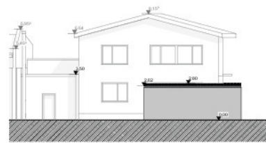
ENDZUSTAND ANSICHT A-06
