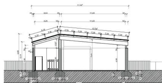
ENDZUSTAND SCHNITT S-01
