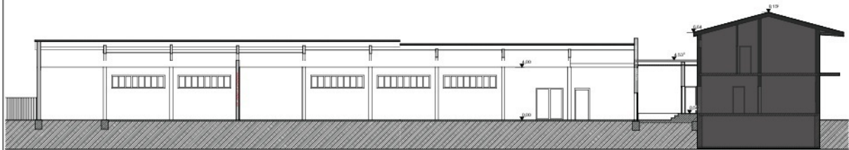
ENDZUSTAND SCHNITT S-02
