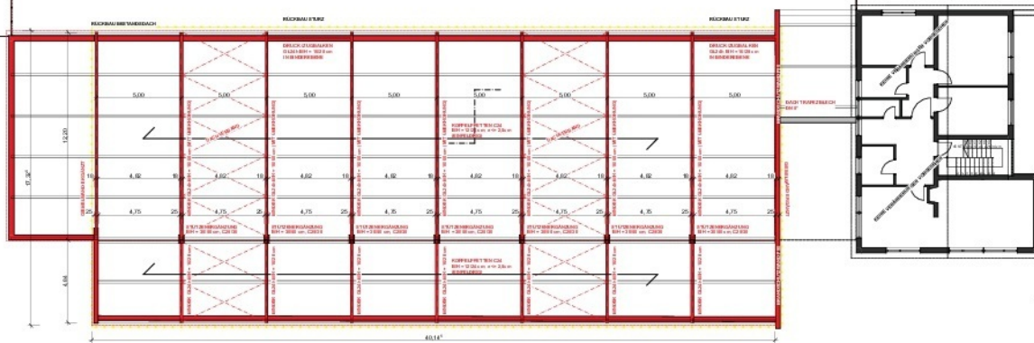
ABBRUCH/NEUBAU GRUNDRISS DACH
