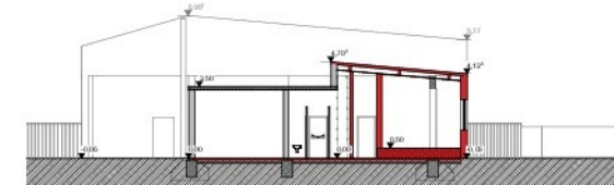
ABBRUCH/NEUBAU SCHNITT S-03
