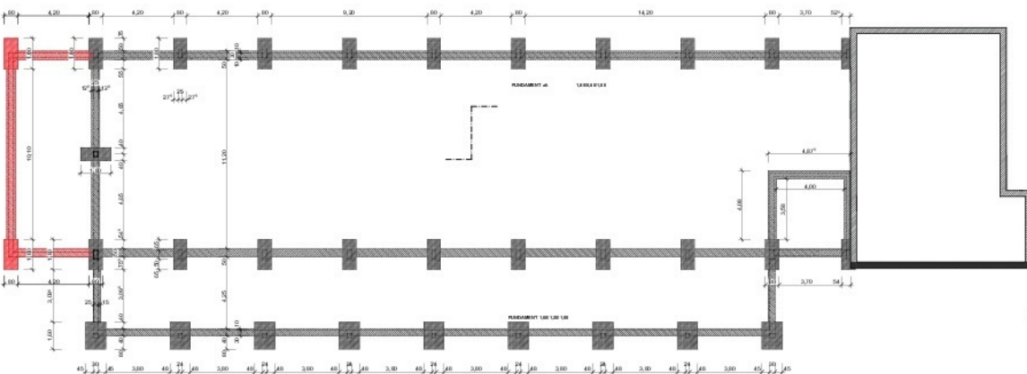
ABBRUCH/NEUBAU GRUNDRISS FUNDAMENTE
