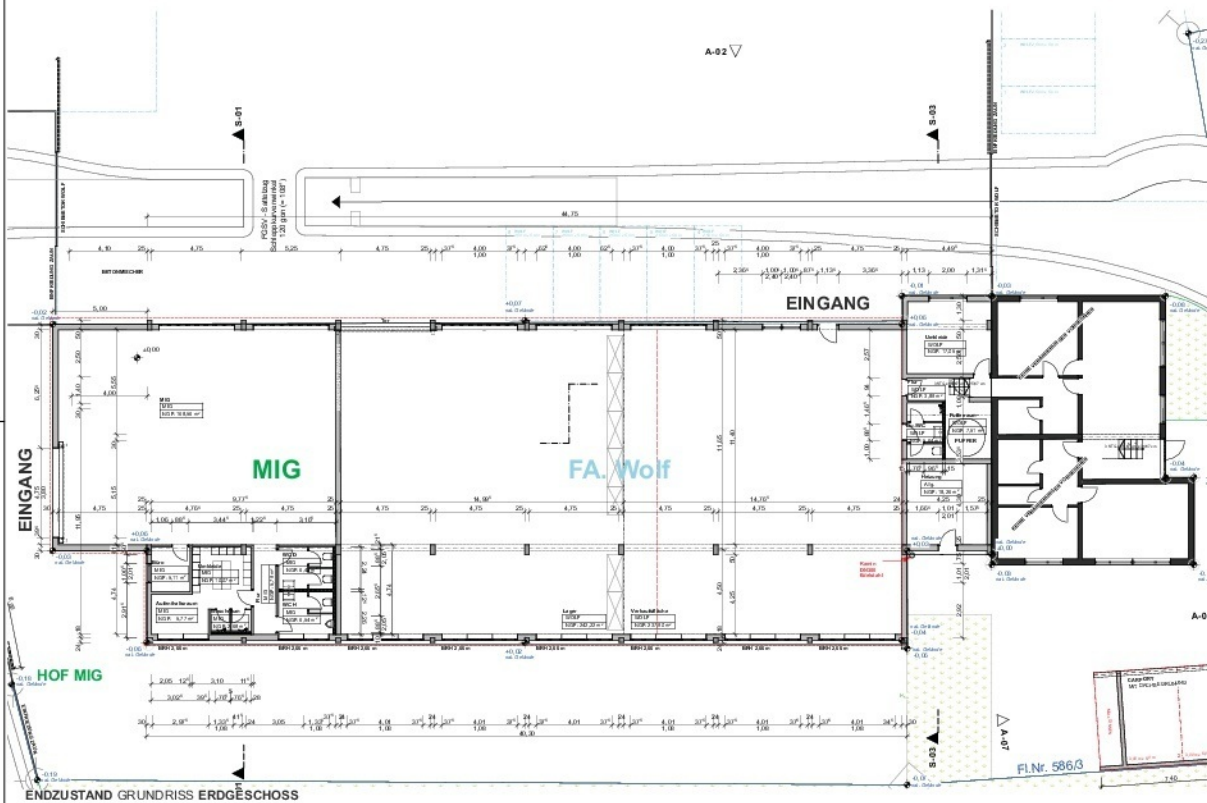
ENDZUSTAND GRUNDRISS ERDGESCHOSS
