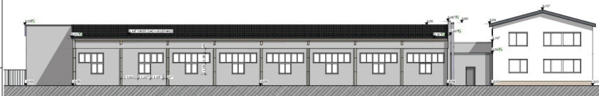
ENDZUSTAND ANSICHT A-03 SÜD-WEST
