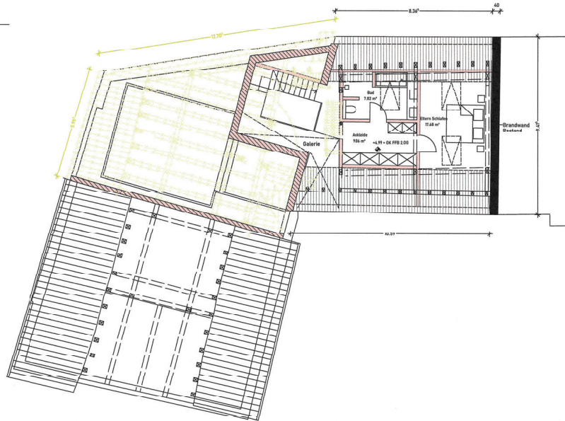
Grundriss 2.OG M 1:100
