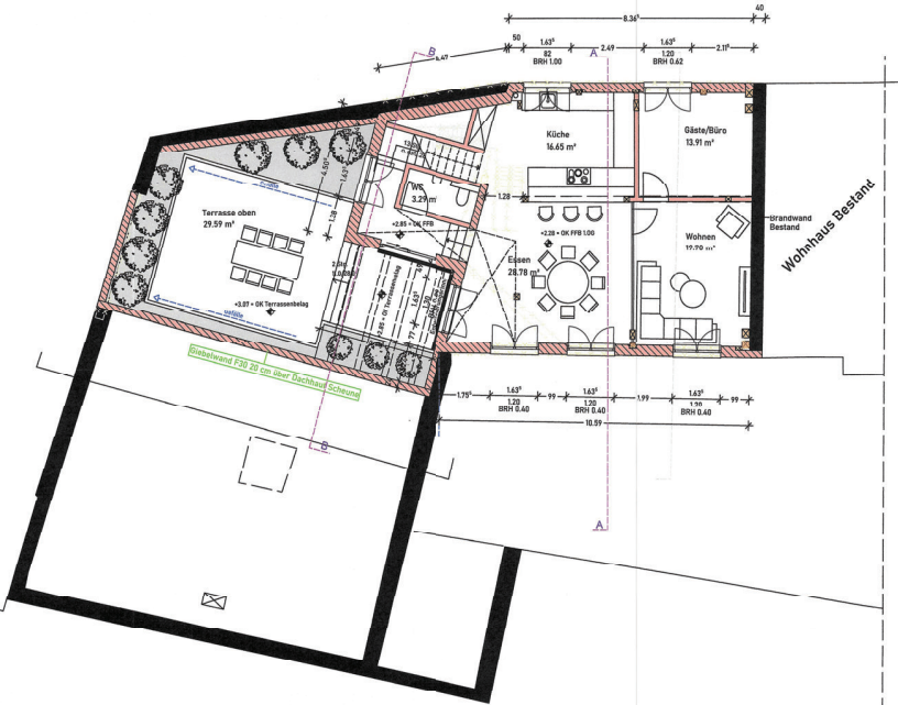
Grundriss 1.OG M 1:100
