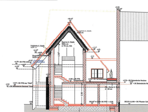
Schnitt B-B M 1:100
