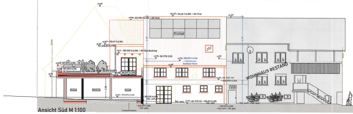
Ansicht Süd M 1:100
