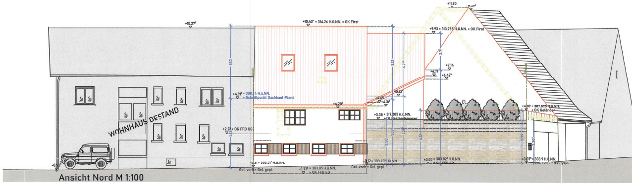
Ansicht Nord M 1:100
