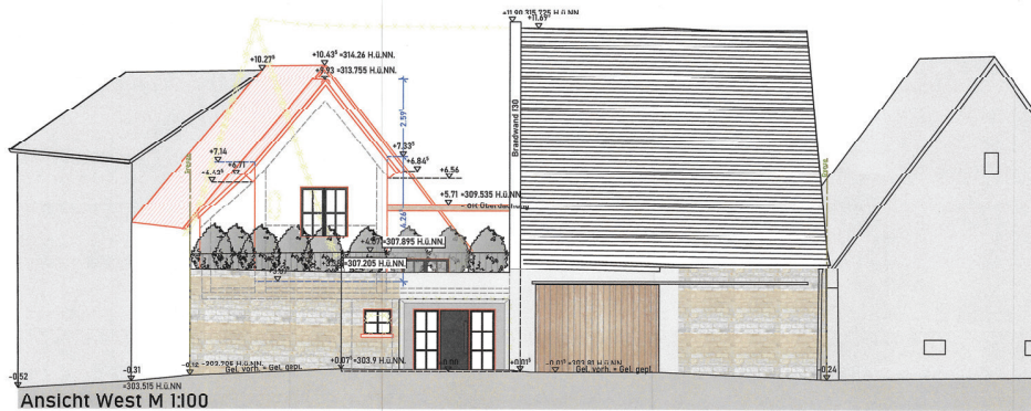
Ansicht West M 1:100
