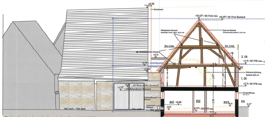
Schnitt A-A mit Ansicht Ost M 1:100
